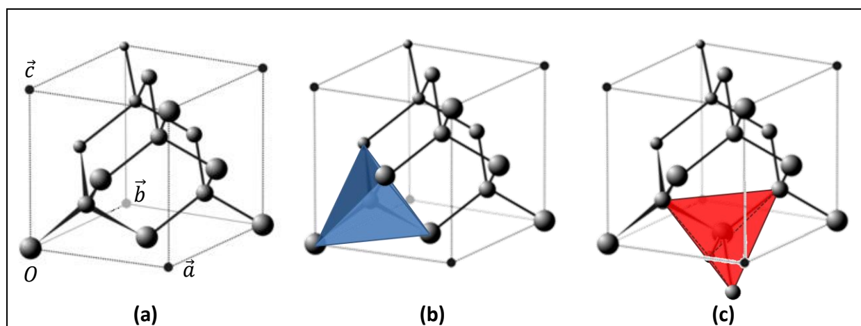
Figure 3 : (a) Rappel de la maille cubique du diamant. En tenant compte de la répétition de la maille dans les 3 directions de l'espace, on peut se convaincre que chaque atome de la structure est en coordination tétraédrique (hybridation sp^3 du carbone). (b) En bleu : représentation du tétraèdre formé par les premiers voisins de l'atome situé en (\frac{1}{4}, \frac{1}{4}, \frac{1}{4}) . Les atomes situés en (\frac{3}{4}, \frac{3}{4}, \frac{1}{4}) , (\frac{3}{4}, \frac{1}{4}, \frac{3}{4}) et (\frac{1}{4}, \frac{3}{4}, \frac{3}{4}) présentent un environnement tétraédrique de même orientation. (c) En rouge : représentation du tétraèdre formé par les premiers voisins de l'atome situé en (\frac{1}{2}, \frac{1}{2}, 0) . Les atomes situés aux sommets et au centre des faces de la maille cubique présentent un environnement tétraédrique de même orientation.
